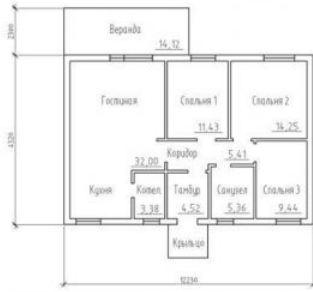
Экспликация помещений
