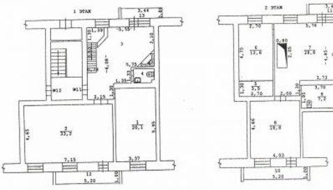
ПЛАН КВАРТИРЫ № 11 (выкопировка из поэтажного плана дома) М 1:200
