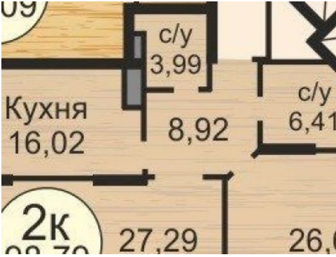
Планировочное решение двухкомнатной квартиры S=98,79м 2
